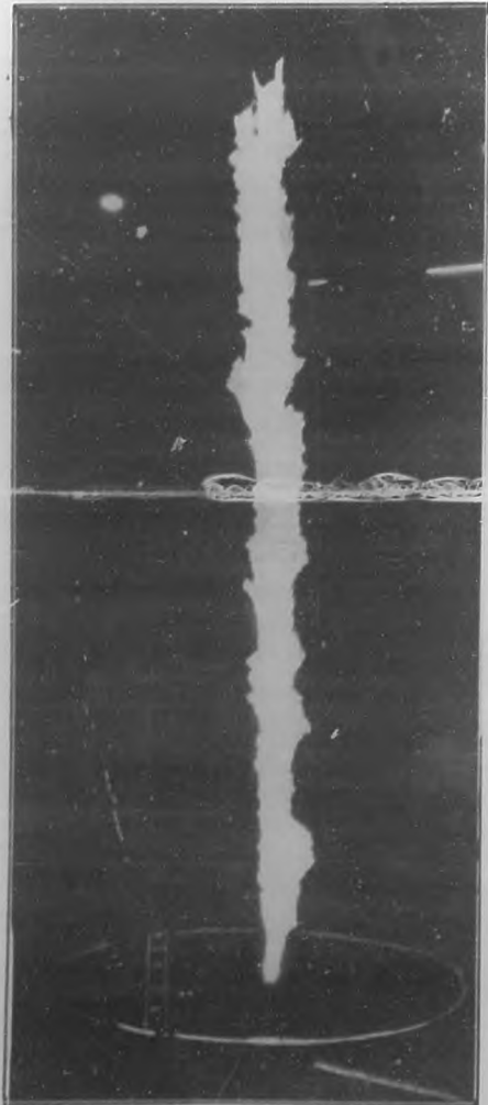
Un arco electrizado de 42 pies de longitud. Experimento realizado en los laboratorios de alto voltaje de la Westinghouse Electric and Manufacturing Co., en Trafford City, Pa., utilizando una corriente de un millón de volts.
